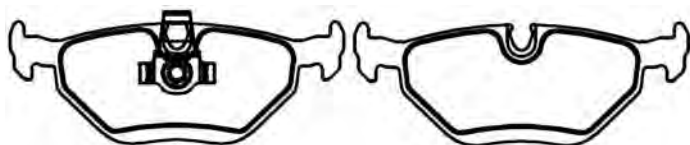
PFC240004 Dimensões em MM: 155,20 x 68,40 x 20,00
