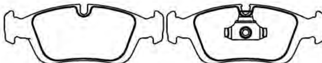
PFC240014 Dimensões em MM: 154,70 x 63,50 x 19,00
