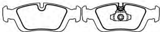
PFC240003 Dimensões em MM: 122,80 x 45,39 x 17,00
