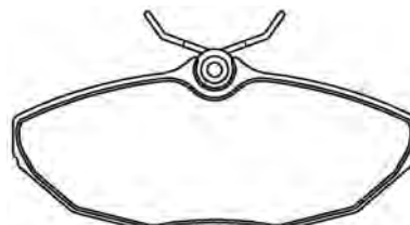
PFC490003 Dimensões em MM: 156,30 x 78,50 x 19,00 Dimensões em MM: 155,10 x 71,40 x 19,00
