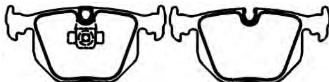
PFC240010 Dimensões em MM: 155,00 x 63,75 x 20,00
