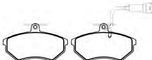
PFC510001 Dimensões em MM: 118,70 x 69,00 x 17,00
