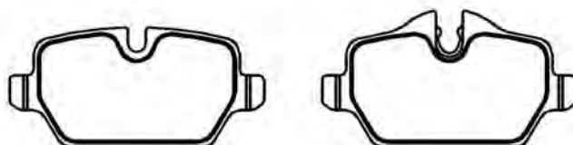
PFC240012 Dimensões em MM: 95,40 x 44,80 x 17,00 Dimensões em MM: 95,40 x 51,20 x 17,00
