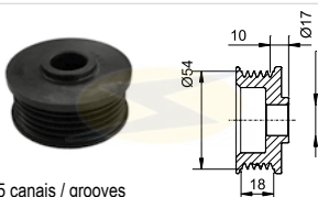
5 canais / grooves
