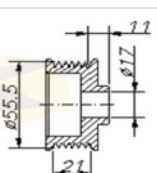
6 canais / grooves
