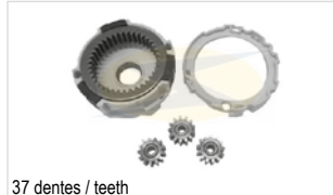
37 dentes / teeth
