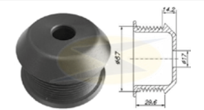
8 canais / grooves
